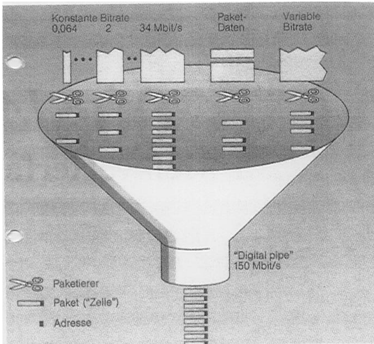
Bild 1. ATM-Prinzip
