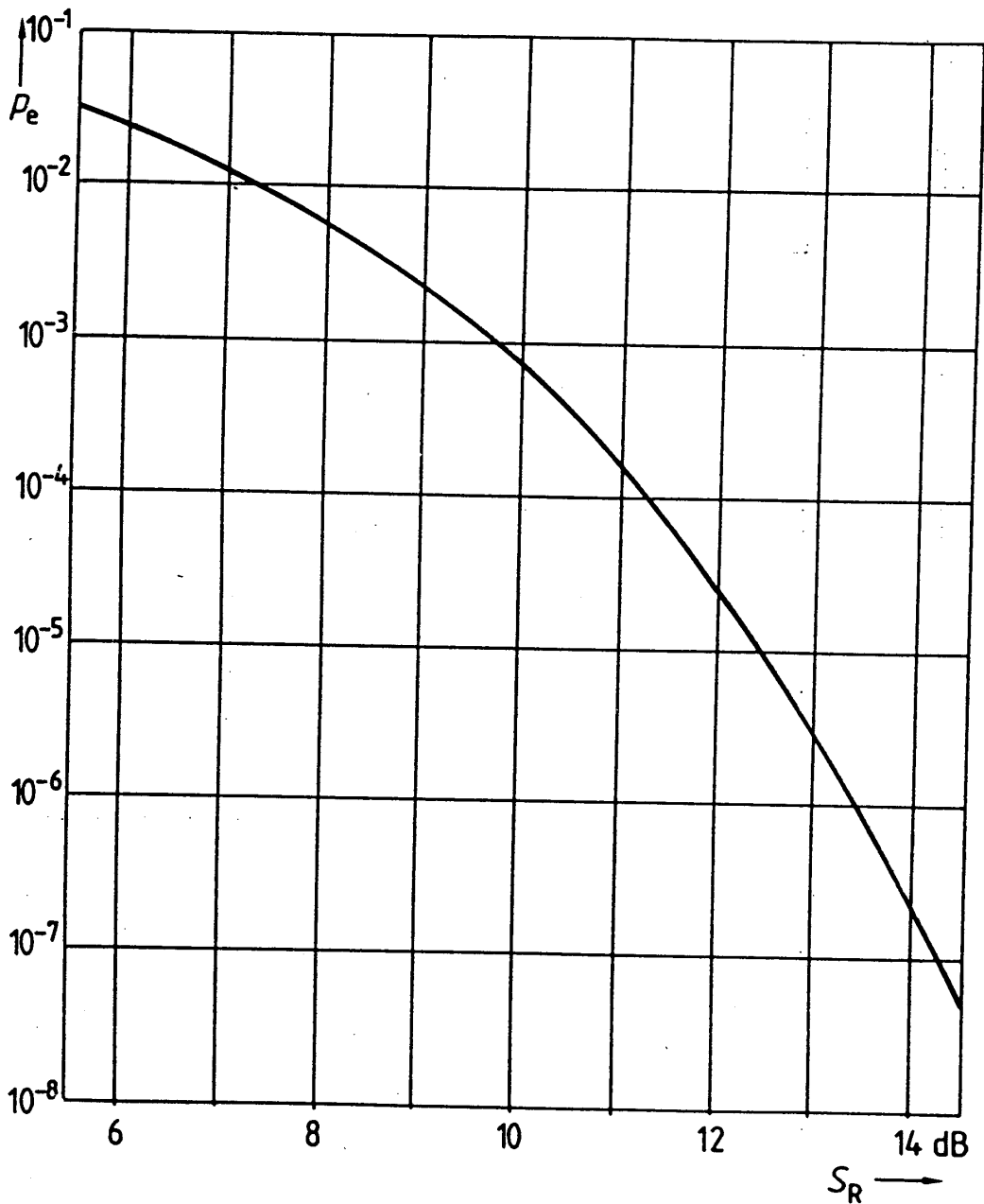
Bild 2.84 Bitfehlerhäufigkeit in Abhängigkeit vom Signal/Rauschabstand im Übertragungskanal mit einem binären NRZ-Rechtecksignal
