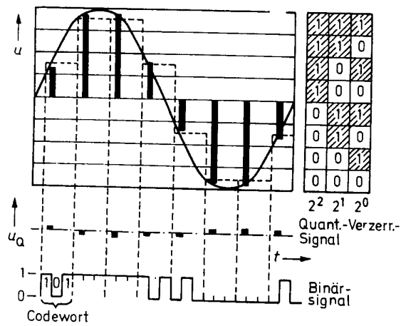
Beispiel für gleichmäßige Amplitudenquantisierung und Codierung mit 3 bit
