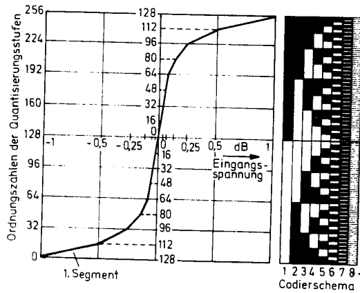
Quantisierungskennlinie 13 Segmente, 8 bit, A-Kurve
