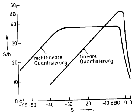
Signal Geräuschabstand bei 8-bit-Codierung
