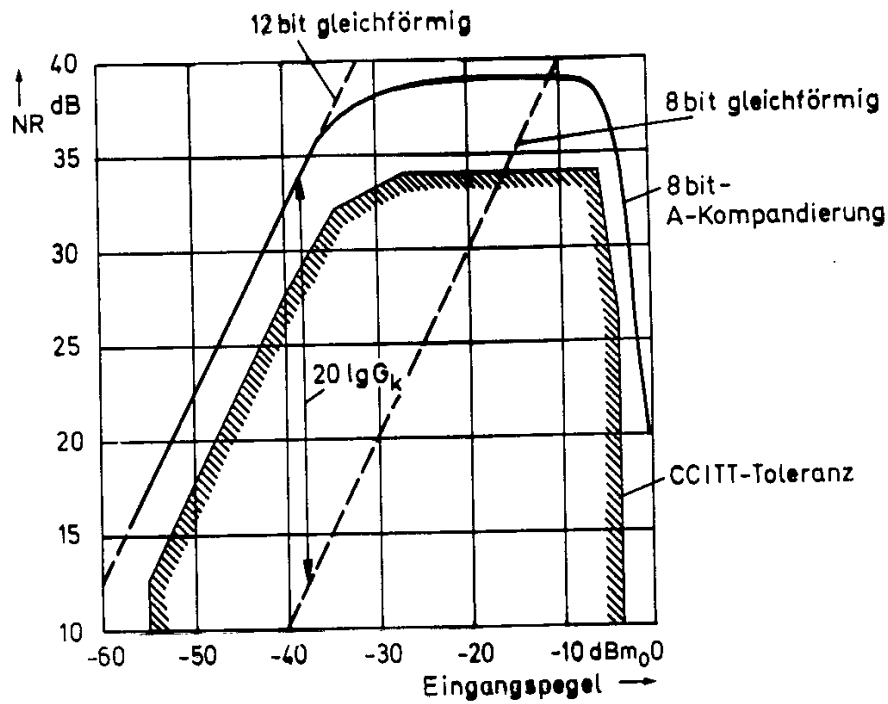
Bild 5.11. Signal-Geräuschverhältnis SNR bei gleichmäßiger und ungleichmäßiger Quantisierung
