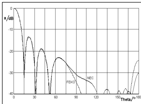
Bild 3: Vergleich der Fernfeldberechnungen (f=900 MHz)
