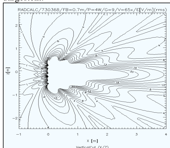
Bild 6: RADCALC-Nahfeld, Einzelmodul mit 65^\circ vertikaler Halbwertsbreite
