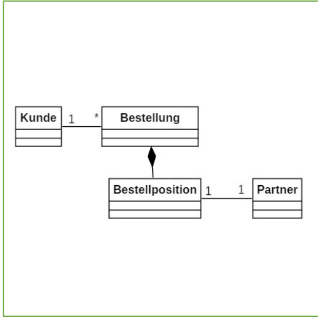
Klassendiagramm
