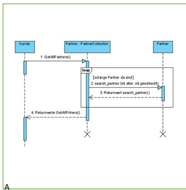
Sequenzdiagramm
