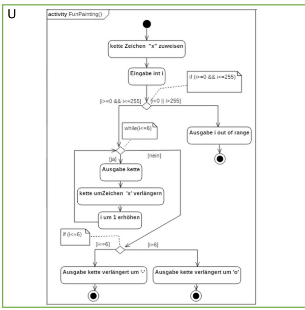
Aktivitätsdiagramm
